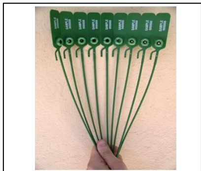
Art: JUPITER SEAL SEAL Sigillo di plastica con chiusura metallo. Coda rotonda, liscia. Con e senza pretaglio Stampa laser. 2 x 315 mm 2 x 425 mm
